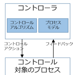
図 2 STAMP モデルの基本構成
