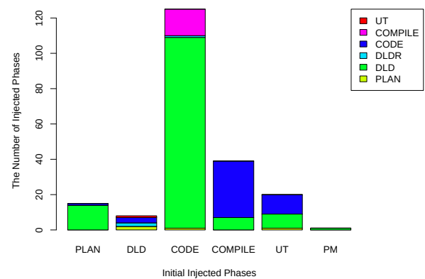
図 17. 修正前の埋込フェーズに対する修正後の埋込フェーズ
