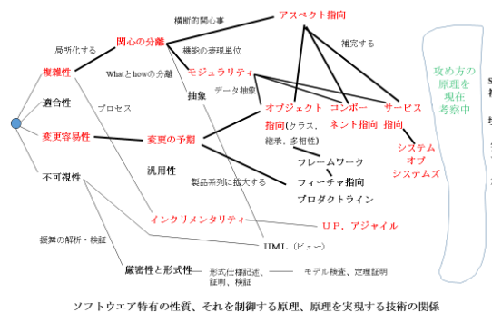
図2 伝統的なソフトウェア工学の成果
